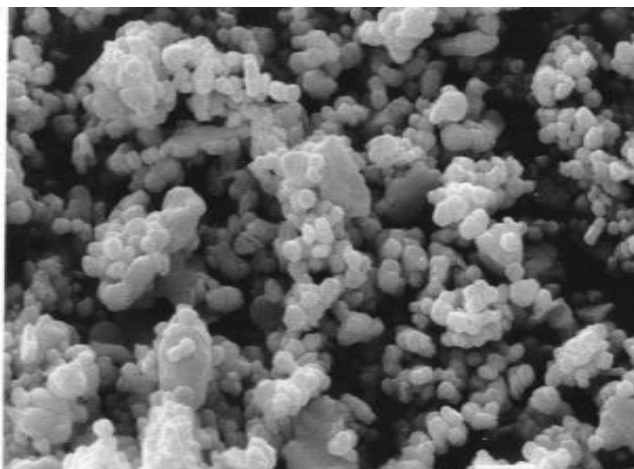
10kx SEM of 70%Ag / 30%Pd AgPd 7558
